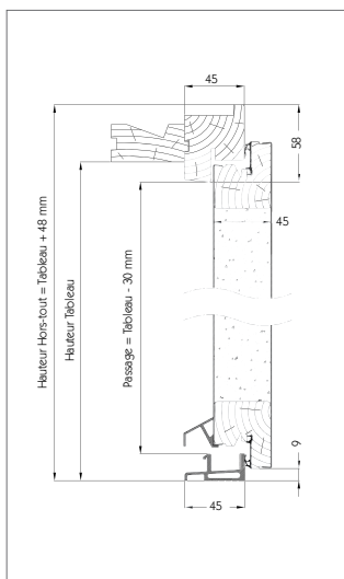
COUPE VERTICALE AVEC DORMANT BOIS
